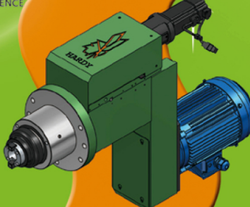
水車伺服鑽孔 / 攻牙動力頭 Servo Drilling / Tapping Spindle Head-Flange Type
