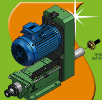
攻牙動力頭 Tapping Spindle Head
