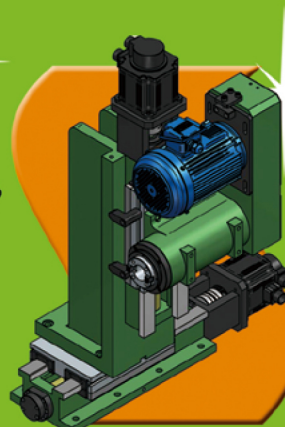
XYZ 三軸伺服滑台 + 搪銑頭 XYZ Servo Slide Table + Milling Head
