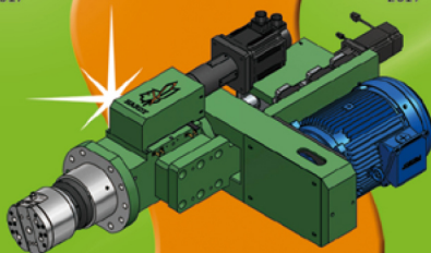
水車式伺服展刀動力頭 Facing Spindle Head-Servo / Flang Type
