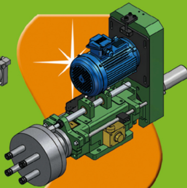
多軸主軸頭 Multi-Spindle Head
